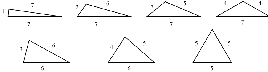
Fig. 1 Die 7 Dreiecke mit Umfang 15
